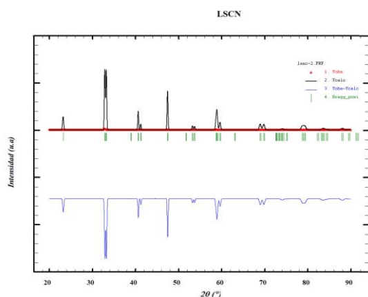
Figura 4. Refinamiento Rietveld empleando los datos de DRX del compuesto LSCN. En la Figura 5, se observa la estructura cristalina obtenida después del refinamiento Rietveld.
