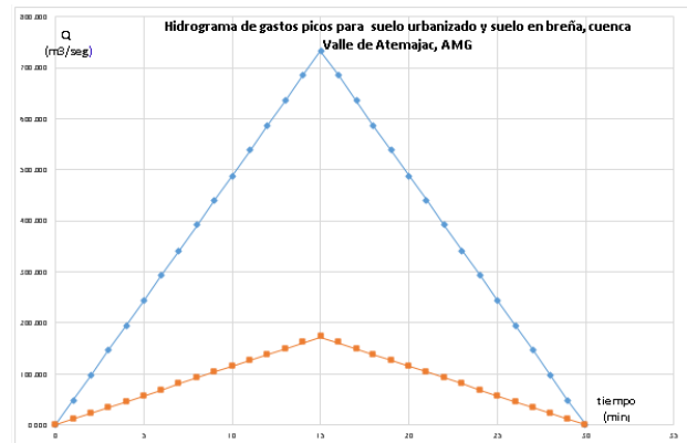
Gráfico 1. Hidrograma de gastos picos para suelo en breña y urbanizado
