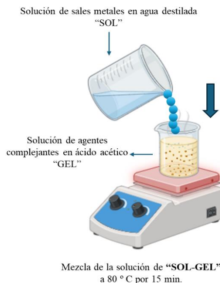
Figura 1. Síntesis del compuesto LSCN mediante el método SOL-GEL vía polimérica.
