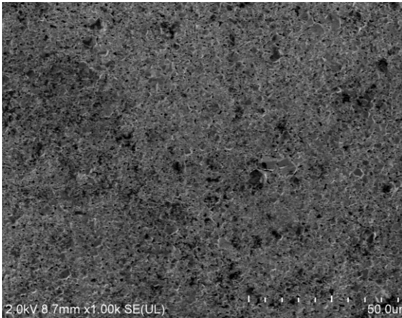
Figura 3 Micrografía obtenida de la muestra de Referencia.
