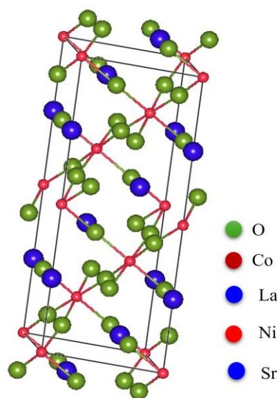
Figura 5. Estructura cristalina obtenida después del refinamiento, enlaces de los átomos de Co con O
