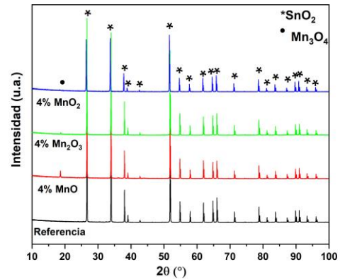
Figura 2 Patrones de difracción para las muestras dopadas con MnO/Mn 2 O 3 /MnO 2 .
