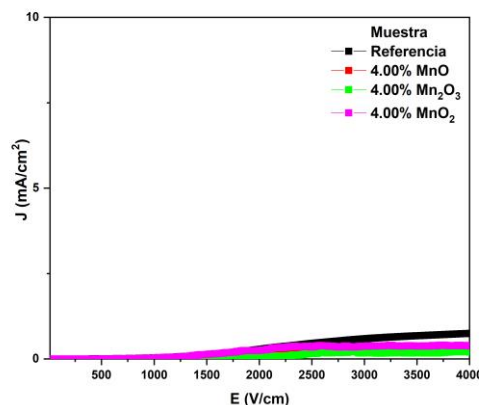
Figura 5 Curvas características J/E.
