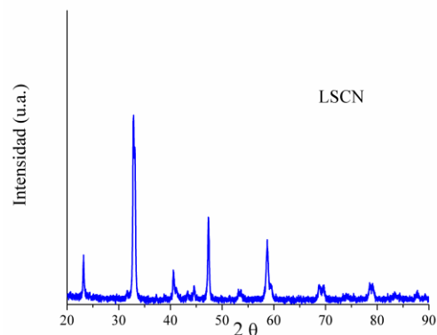
Figura 3. Difracción de rayos X del compuesto
